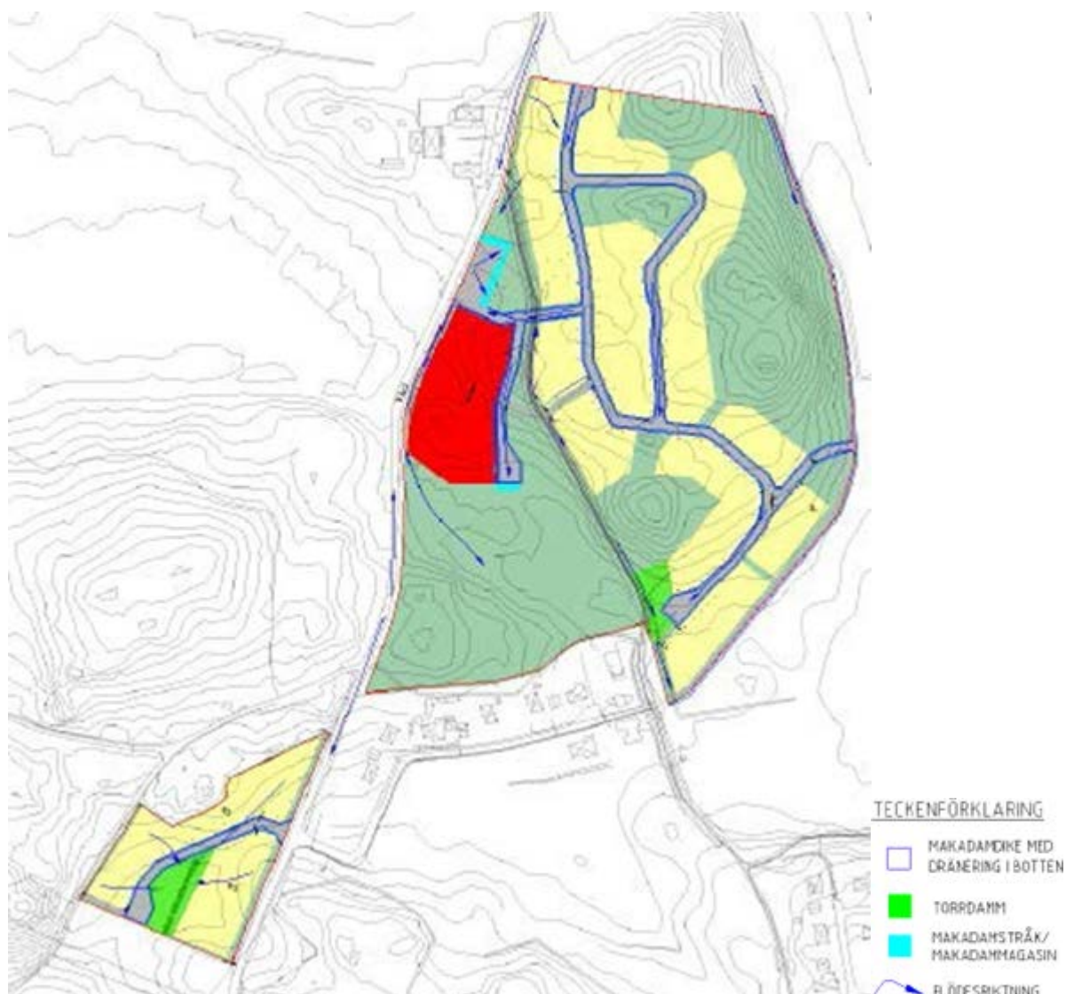
Figur 13. Avvattningsplan med föreslagen dagvattenhantering. Ett makadamdikessystem leder dagvatten till den lågpunkt som ligger närmast nedströms.
