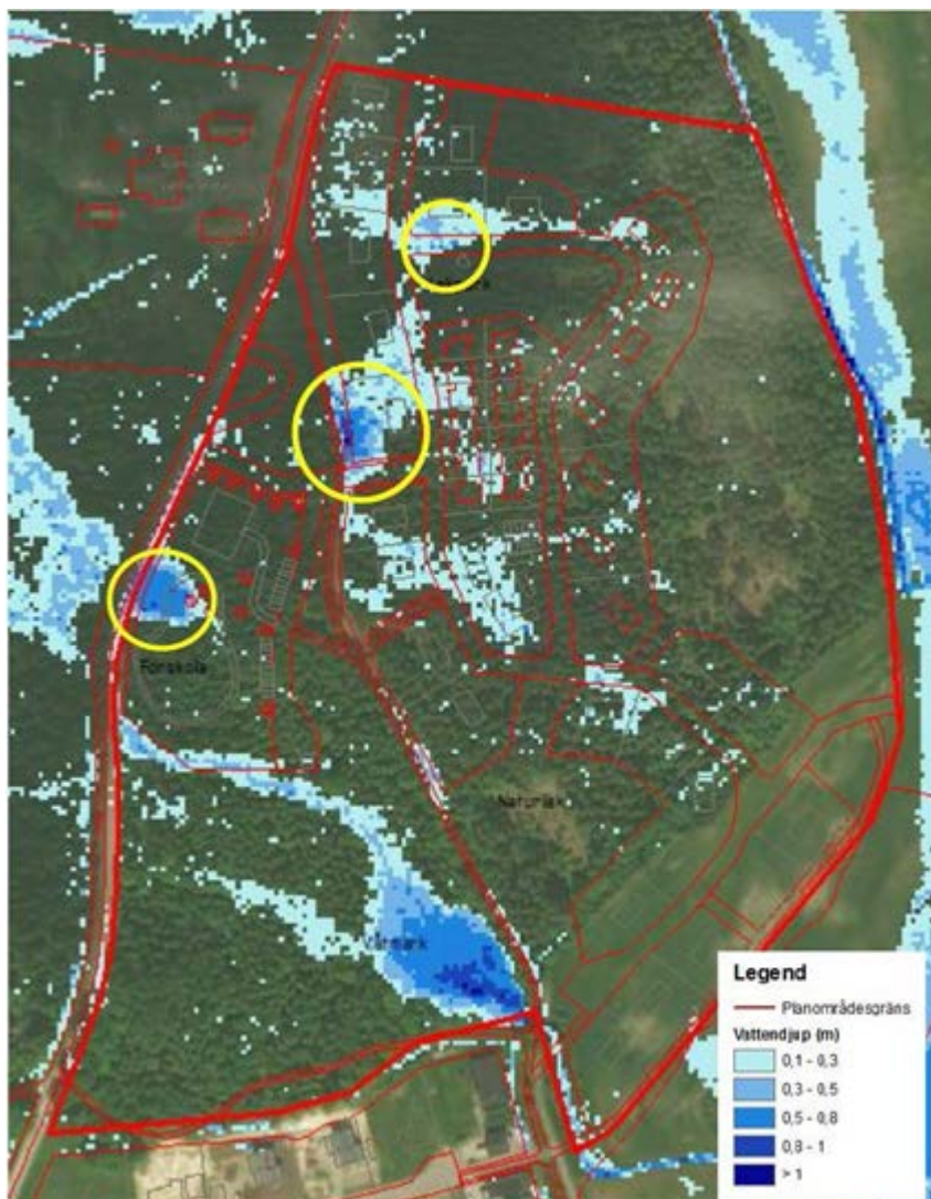
Figur 14. Modellerat maximalt översvämningsdjup i detaljplaneområdets norra del. Tre potentiellt problematiska områden är inringade med gult. Fastighetsgränser i rött.
